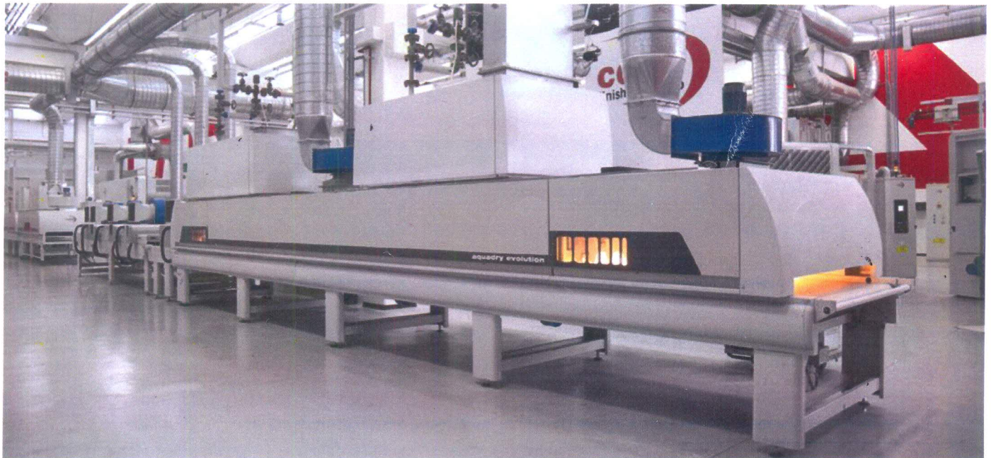
CEFLA UV LACQUER MACHINE
